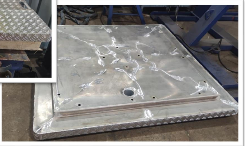
Puertas estancas y escotillas en acero al carbón, acero inox. y aluminio.
