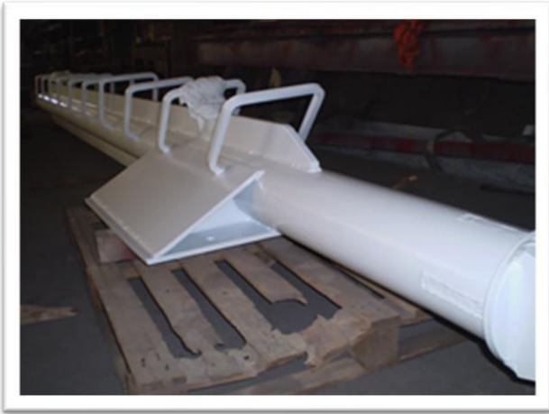
Construcción de plumas para un atunero.
