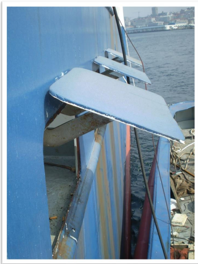
Ventana practicable para visión cofa.
